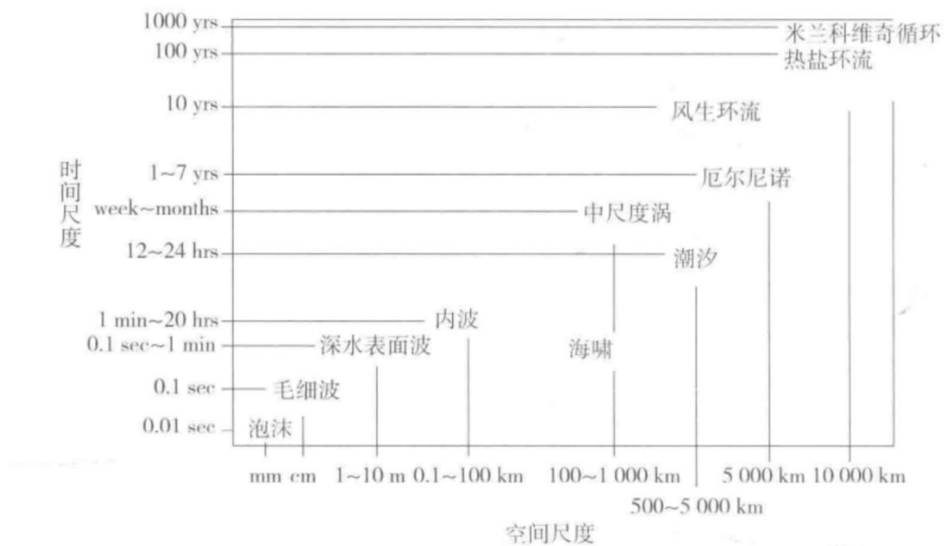
图 1.2 物理海洋学现象(从泡沫和毛细波至大洋环流等)的时间和空间尺度
